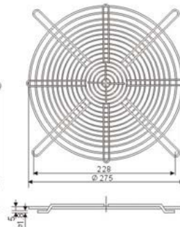
JL-250 FOR 250MM FAN
