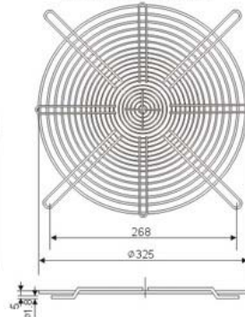
JL-300 FOR 300MM FAN
