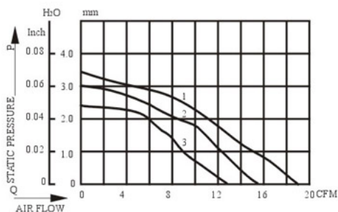
BRUSHLESS FAN 50 × 50 × 15mm
